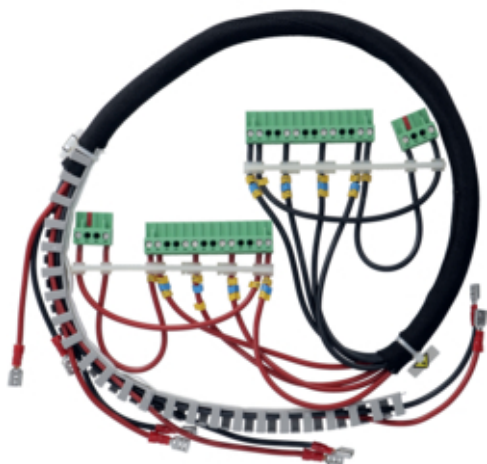
Kit prise de tension commut.1250A
