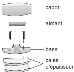
Fig. C - Montage porte-aimant
