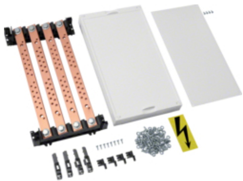
Kit, UniversN, 450x250, jeu de barres 50mm
