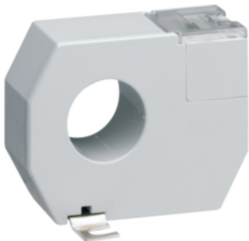
Tore circul \varnothing 210 relais HR5xx
